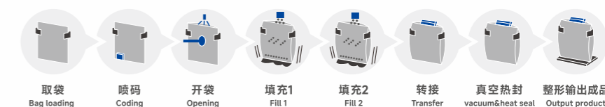
三边封袋 3 side seal bag
