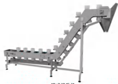
碗式提升机 Bowl lifter
